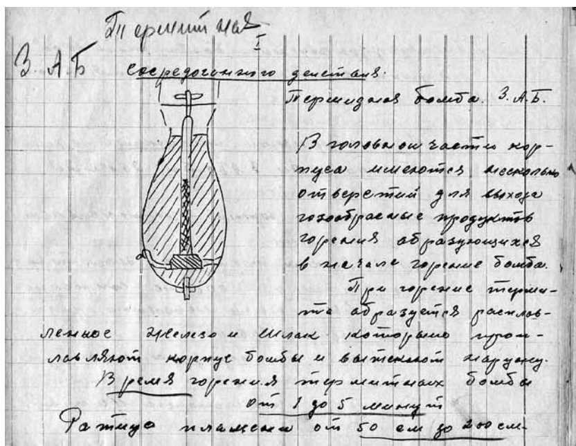
Устройство электронно-термитной зажигательной авиационной бомбы. Конспект, 1942 г.
